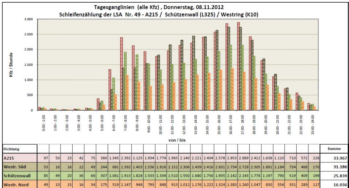
Bild 2.3: Tagesganglinien, Do., 08.11.2012
