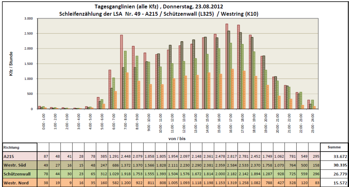
Bild 2.2: Tagesganglinien, Do., 23.08.2012
