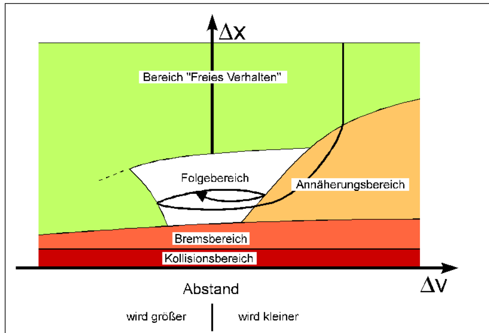
Bild 7.1: Fahrzeugfolgmodell nach Wiedemann (1974)
