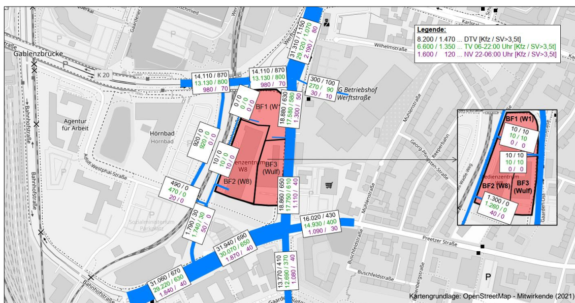
Abbildung 12: P0-Fall 2025 B-Plan 1030V – DTV-Werte (Querschnittbelastungen)
