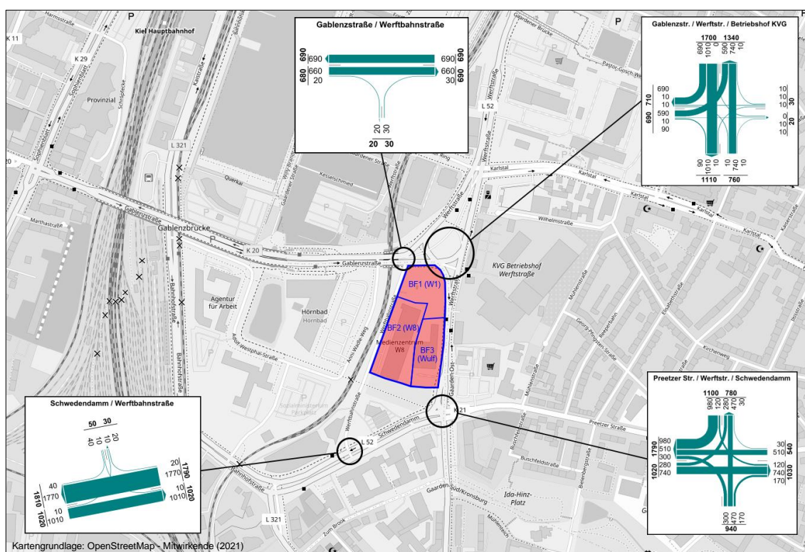
Abbildung 9: Analyse 2019 (2021) – Knotenpunktbelastungen Spitzenstunde spät (in Kfz/h)
