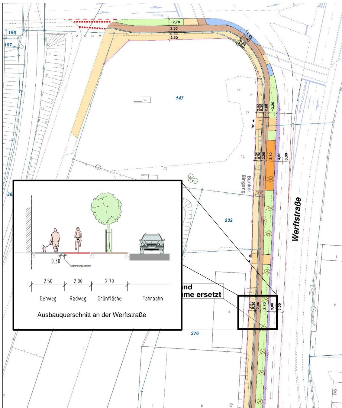
Abbildung 25: Ausbauplanung der Nebenflächen in der Wertstraße – Ausschnitt [24] mit Darstellung des empfohlenen Ausbauquerschnitts
