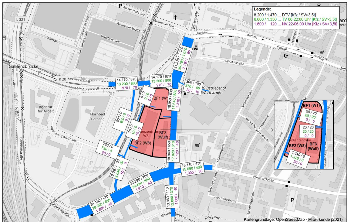
Abbildung 17: Prognoseplanfall 2025 B-Plan 1030V – DTV-Werte (Querschnittbelastungen)
