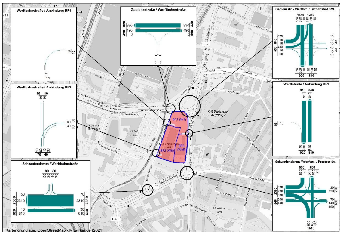
Abbildung 13: P0-Fall 2025 B-Plan 1030V – Knotenpunktbelastungen Spitzenstunde früh (in Kfz/h)
