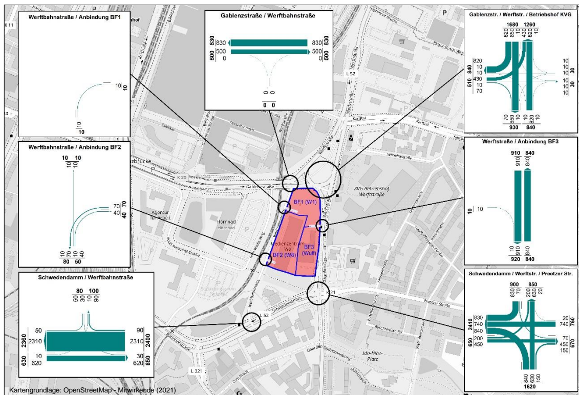
Abbildung 18: Prognoseplanfall 2025 B-Plan 1030V – Knotenpunktbelastungen Spitzenstunde früh (Kfz/h)
