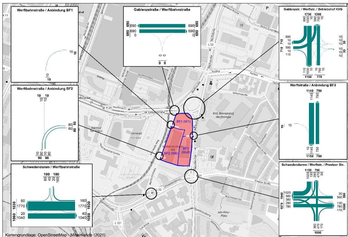
Abbildung 14: P0-Fall 2025 B-Plan 1030V – Knotenpunktbelastungen Spitzenstunde spät (in Kfz/h)
