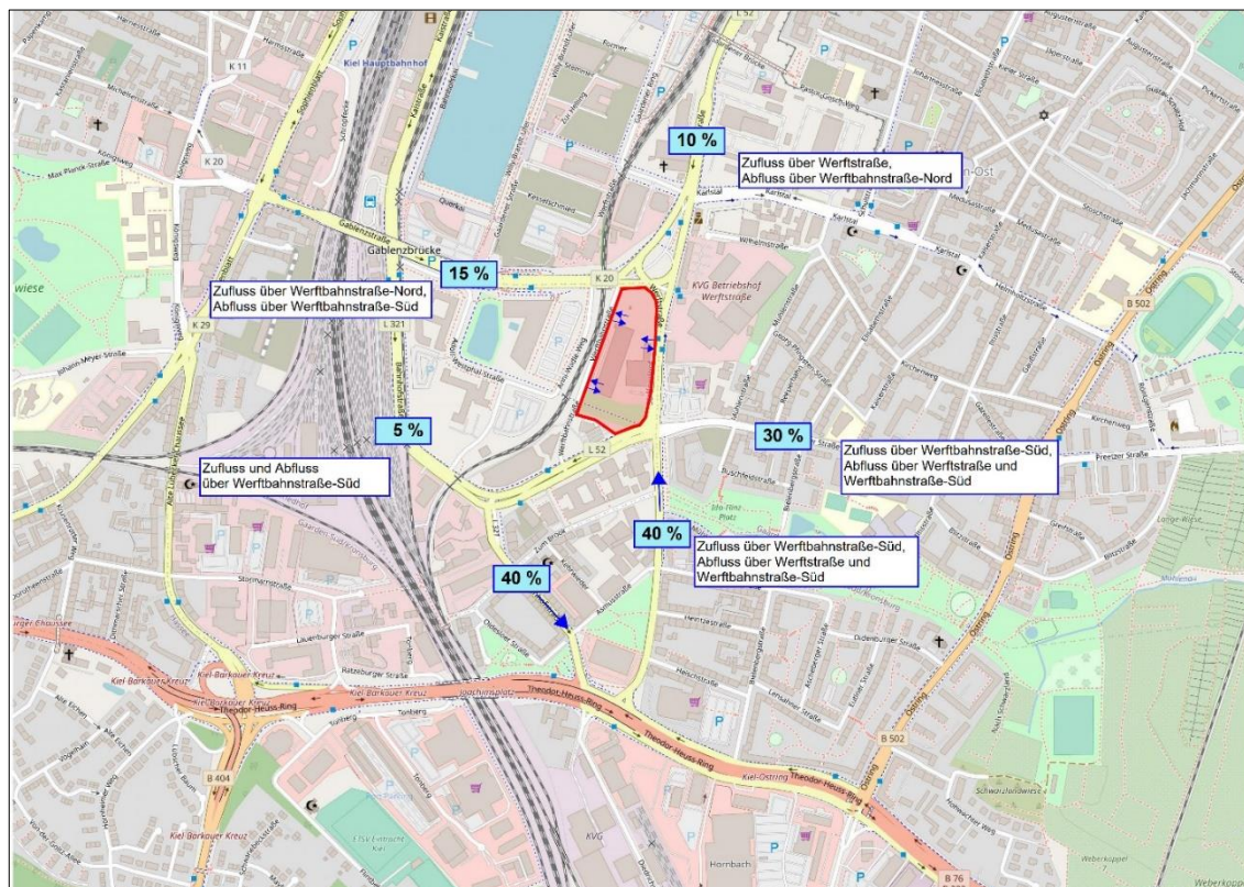
Abbildung 16: Regionale Richtungsverteilung des Kfz-Neuverkehrs B-Plan 1030V
