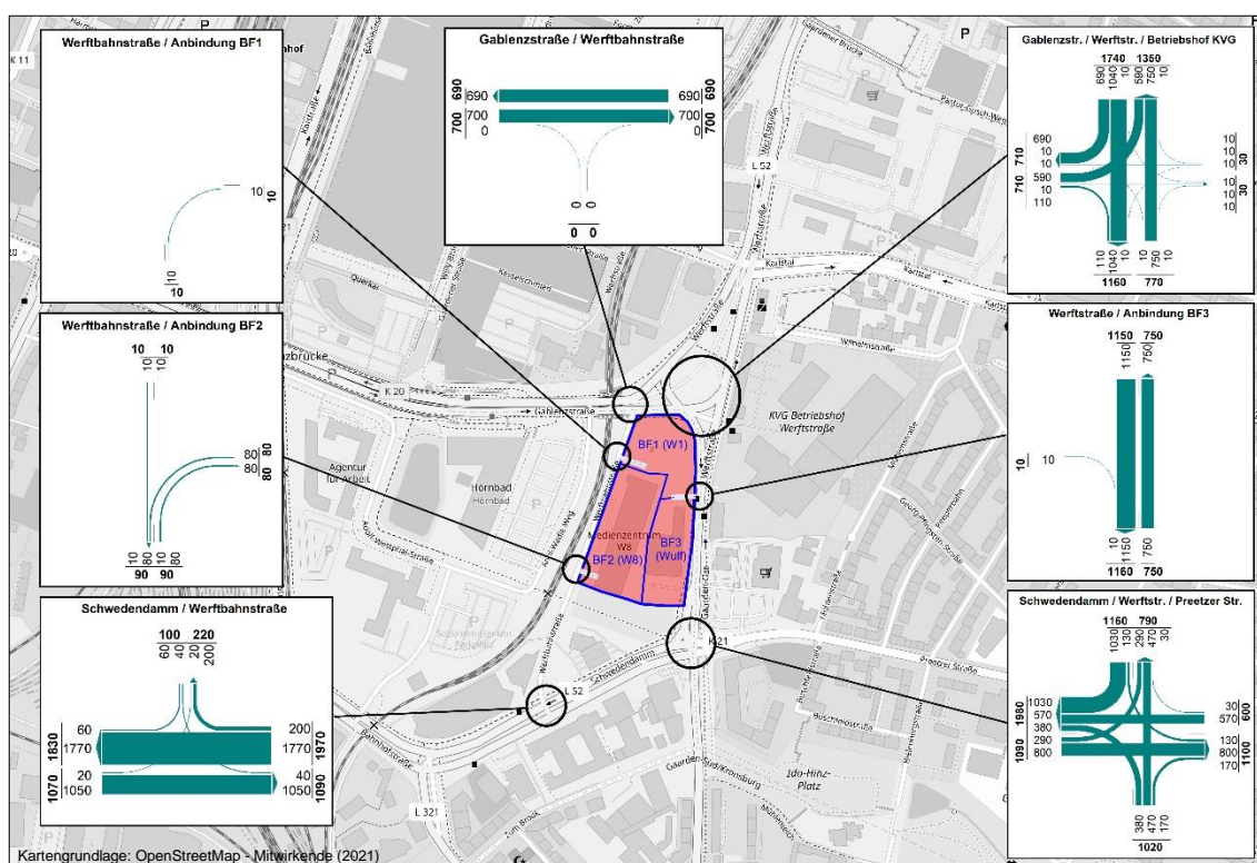
Abbildung 19: Prognoseplanfall 2025 B-Plan 1030V – Knotenpunktbelastungen Spitzenstunde spät (Kfz/h)
