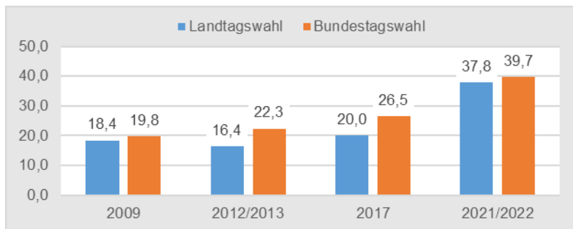
Grafik 1. Briefwähler*innenanteil bei Bundes- und Landtagswahlen seit 2009 in Kiel
