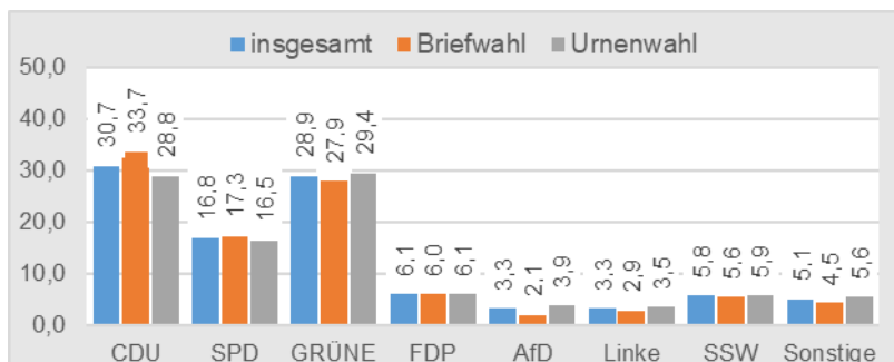
Grafik 2. Zweitstimmenanteile nach Brief- und Urnenwahl bei der Landtagswahl 2022 in Kiel
